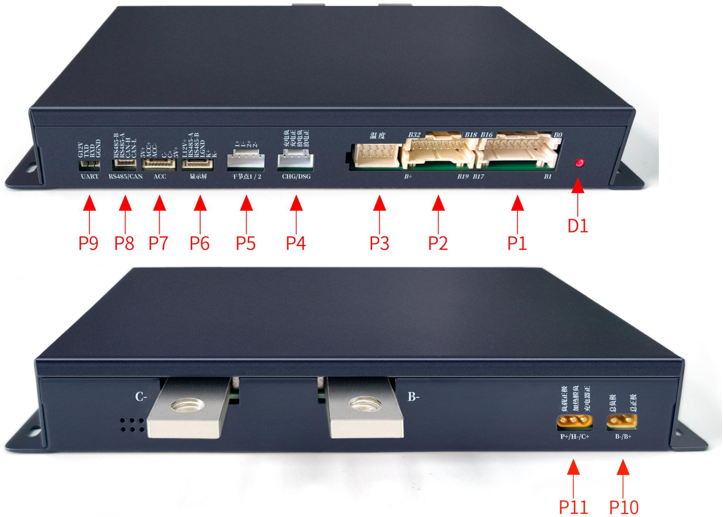
JK-B2A32S-RP 连接器示意图
